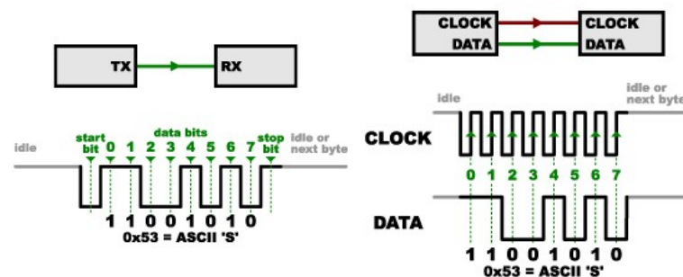
Obr. 74 Časový priebeh asynchrónnej komunikácie(vľavo) a synchronnej komunikácie (vpravo)
