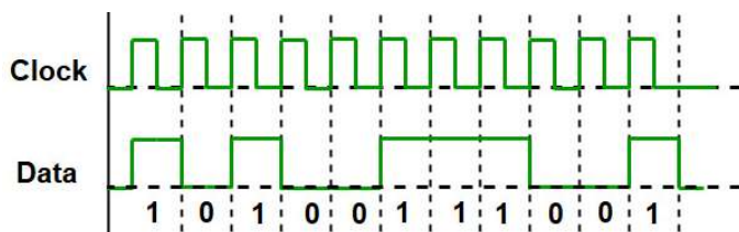
Obr. 3 Synchronizovanie binárnych dát s hodinovým impulzom
