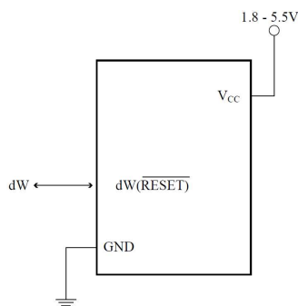
Obr. 90 Schéma prepojenia /RESET vývodu MCU na debugWIRE
