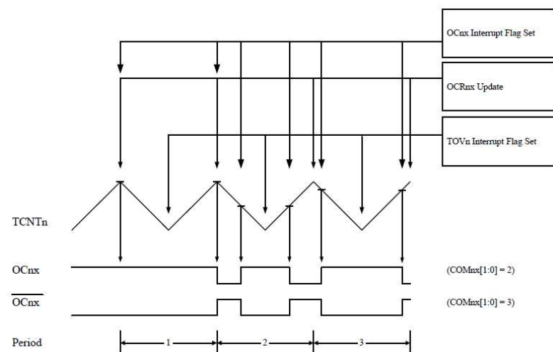
Obr. 70 Časový priebeh zmeny OCn v režime fázovo korektnej PWM
