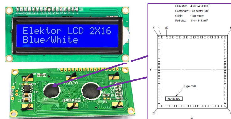
Obr. 93 LCD znakový modul displeja s 2x16 znakov
