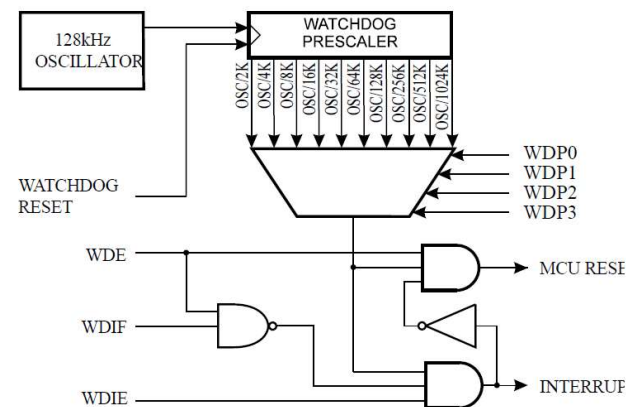
Obr. 46 Bloková schéma WatchDog timer
