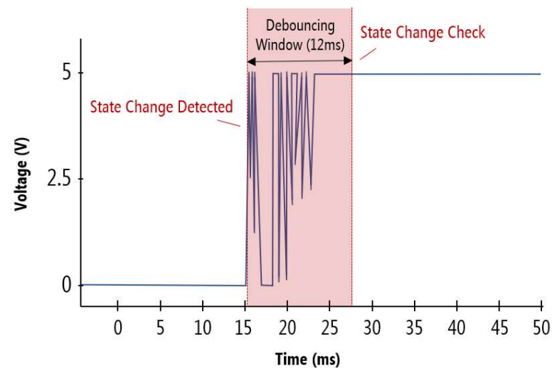
Obr. 15 Príklad softvérové riešenia zákmitov kontaktu pomocou časového okna
