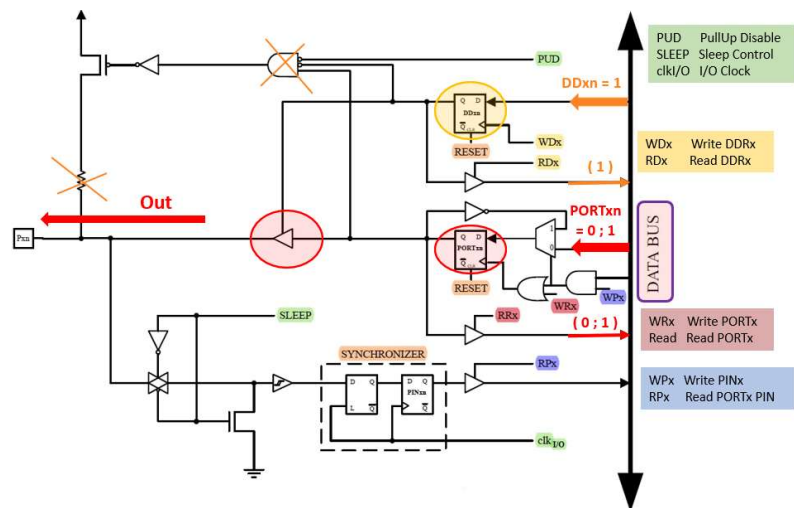
Obr. 51 Logika I/O vývodu v režime výstup (DDxn=1)
