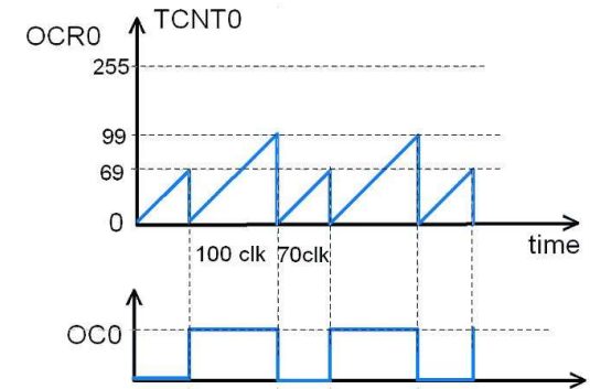
Obr. 62 Příklad priebehu signálu na výstupe OC0A v CTC móde TC0
