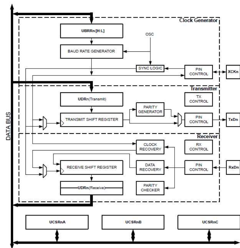
Obr. 79 Bloková schéma USARTu
