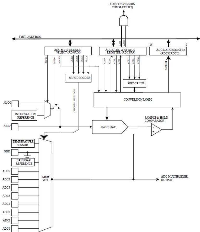
Obr. 88 Bloková schéma A/D prevodníka
