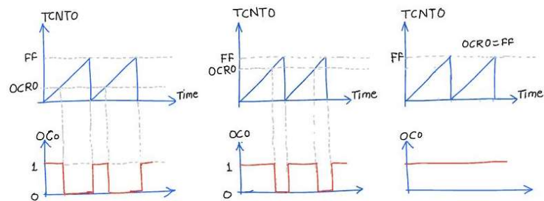
Obr. 64 Jednoduché znázornenie neinvertujúceho Fast PWM signálu
