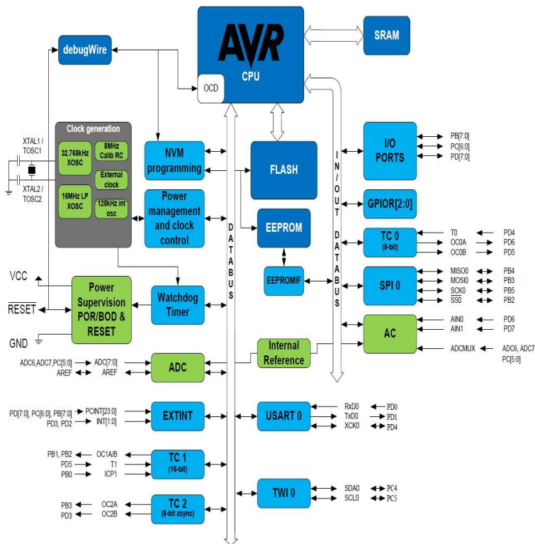
Obr. 36 Bloková schéma ATmega328
