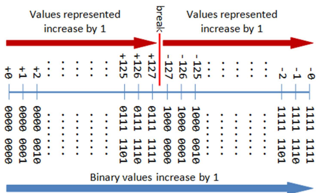
Obr. 17 Kódovanie binárnych čísel jednotkovým doplnkom
