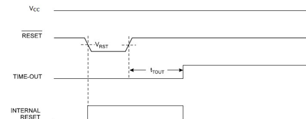
Obr. 43 Časový priebeh External Reset
