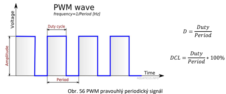
Obr. 56 PWM pravouhlý periodický signál
