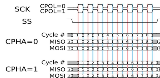
Obr. 77 Časový diagram polaritu a fázu hodinového signálu SPI prenosu.
