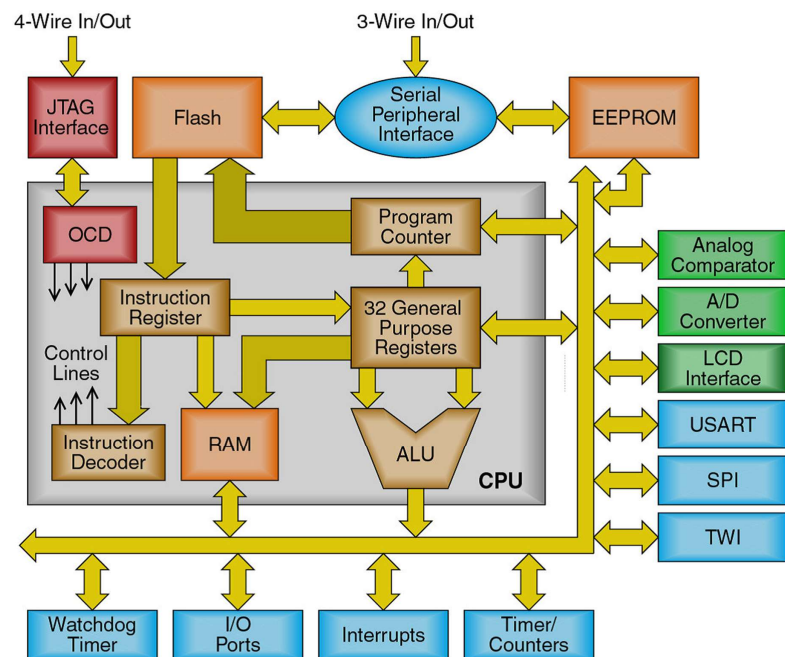
Obr. 31 Bloková schéma AVR mikrokontrolérov
