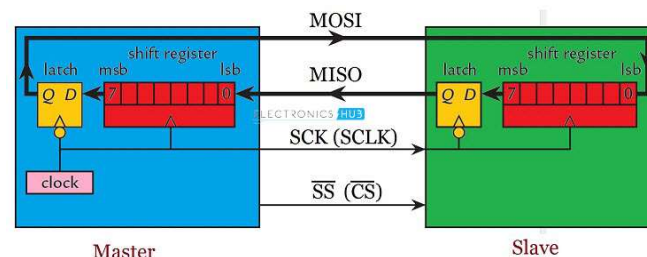
Obr. 76 Hardvérové riešenie duplexného prenosu SPI
