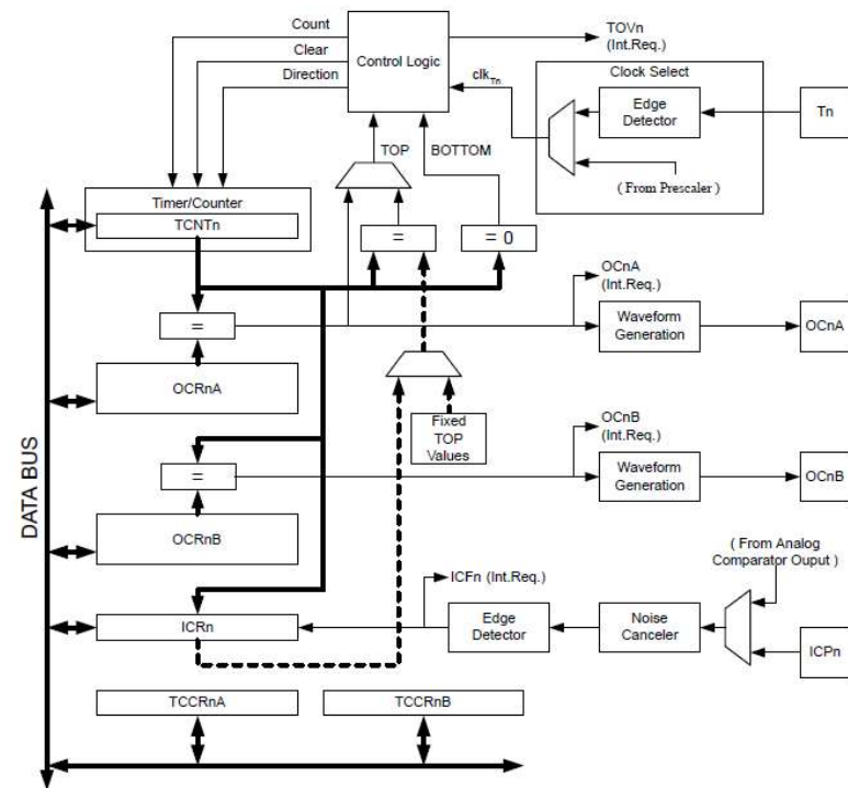
Obr. 72 Bloková schéma 16 bitového časovača – počítača TC1
