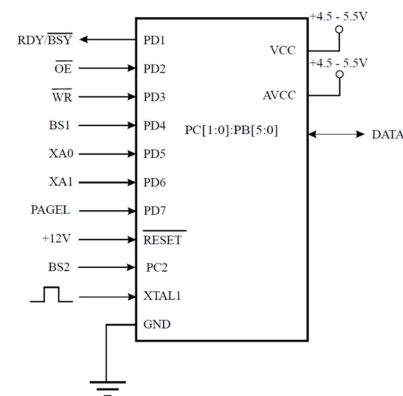
Obr. 30 Schéma zapojenia signálov pre paralelné programovanie
