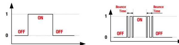
Obr. 10 Signál mechanického kontaktu: a) ideálny, b) reálny
