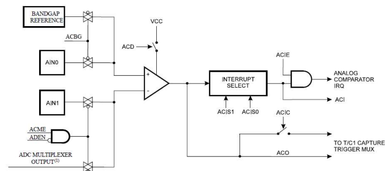
Obr. 89 Bloková schéma logiky AC komparátora
