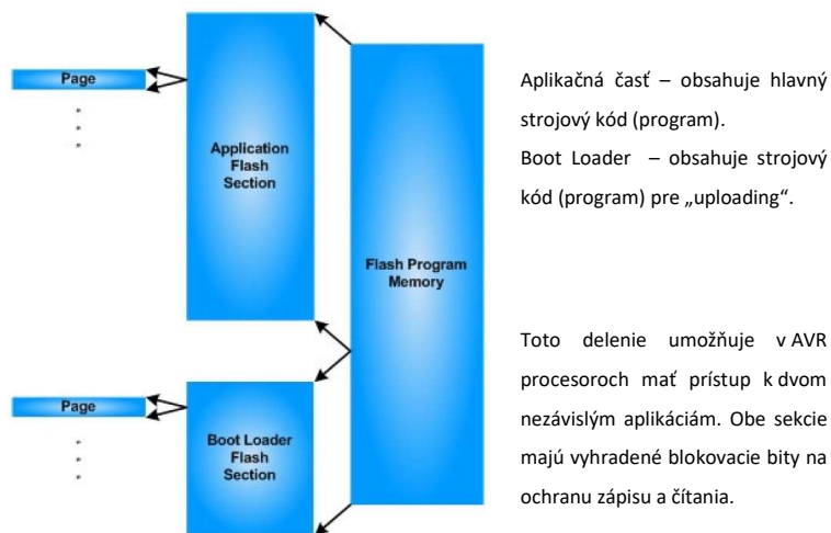
Obr. 28 Rozdelenie programovej Flash pamäte v AVR
