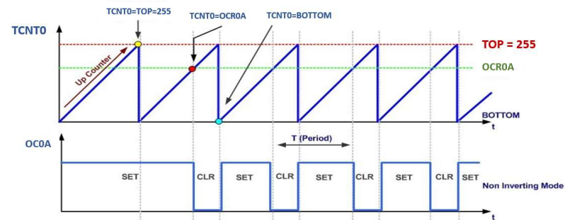
Obr. 66 Příklad časového priebehu zmeny výstupu OC0A v režime Fast PWM
