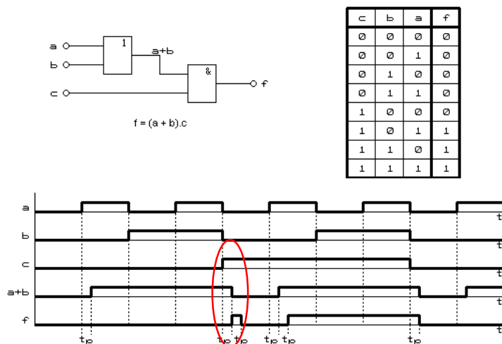
Obr. 9 Príklad vzniku hazardu prechodom signálov logickými obvodmi
