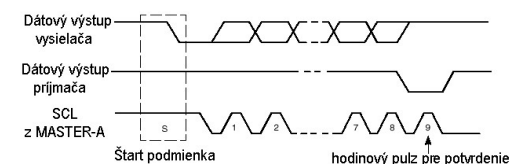
Obr. 86 Potvrdenie prijmu dát ACK zariadením na I2C zbernici
