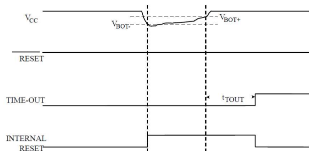
Obr. 44 Časový priebeh Brown-out Reset
