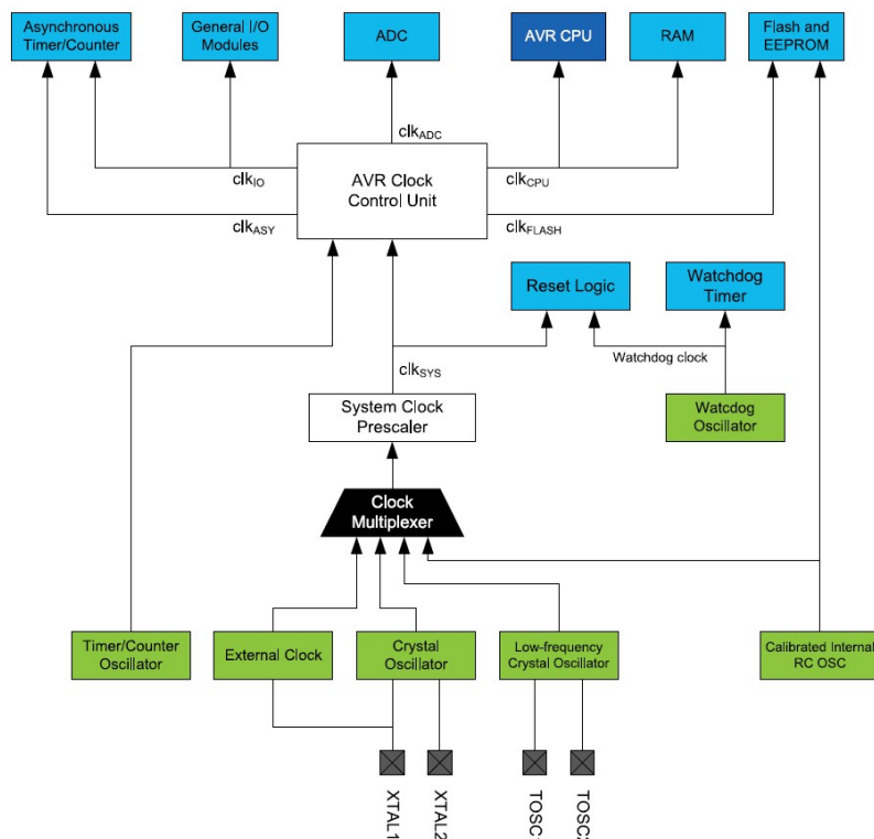
Obr. 38 Zdroje a rozvod hodinového signálu
