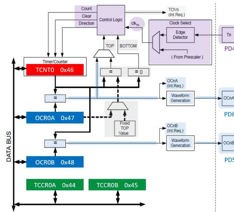
Obr. 58 Bloková schéma TC0 – 8 bitový časovač / počítadlo
