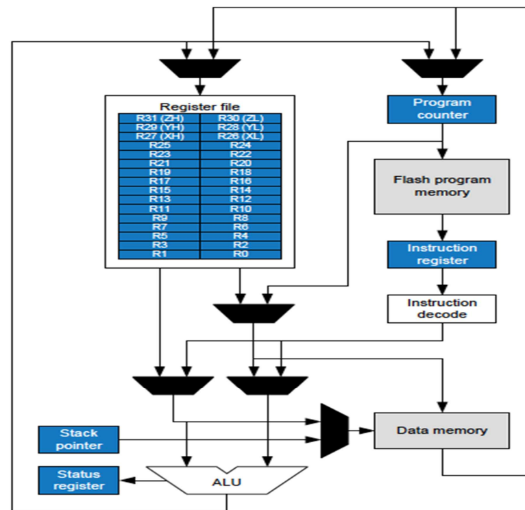
Obr. 21 Bloková schéma jadra AVR
