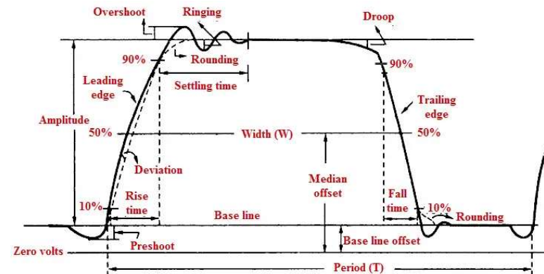
Obr. 4 Parametre digitálneho impulzu
