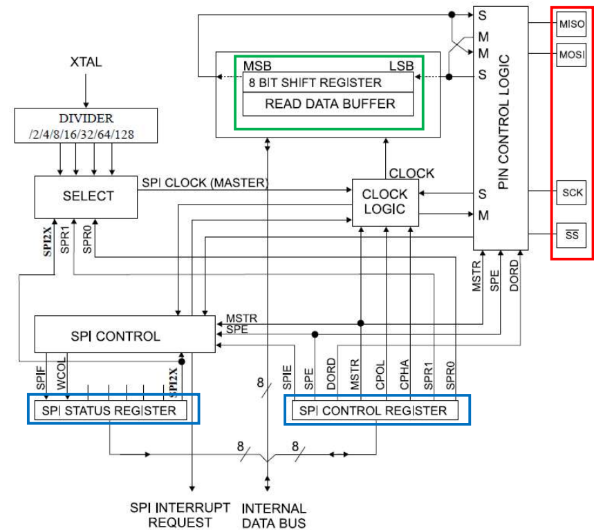
Obr. 78 Bloková schéma SPI v AVR
