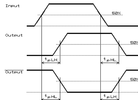
Obr. 8 Prechodové oneskorenie
