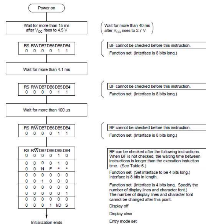
Obr. 99 Postup inicializácie 4-bitového komunikačného prenosu
