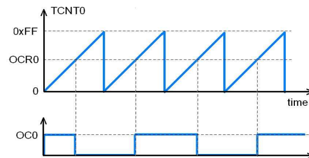
Obr. 60 Priebeh signálu na výstupe OC0A v normálnom móde TCO
