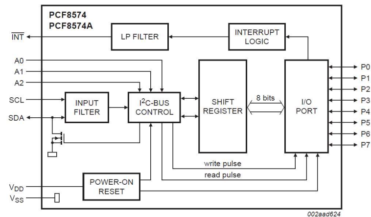
Obr. 102 Bloková schéma PCF8574/74A
