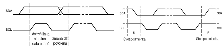
Obr. 84 Funkcia hodinového signálu
