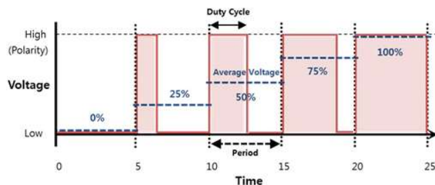
Obr. 57 Princíp generovania regulačného napätia PWM signálom
