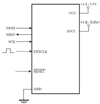
Obr. 27 Schéma zapojenia signálov pre sériové programovanie
