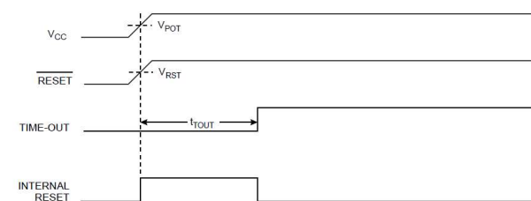
Obr. 42 Časový priebeh Power-on Reset
