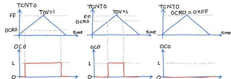
Obr. 69 Jednoduché znázornenie invertujúceho Phase Correct PWM signálu
