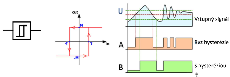
Obr. 14 Schmittov preklápací obvod
