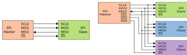
Obr. 75 Zapojenie SPI zbernice (vľavo jedno SPI zariadenie, vpravo viaceré SPI zariadenia)
