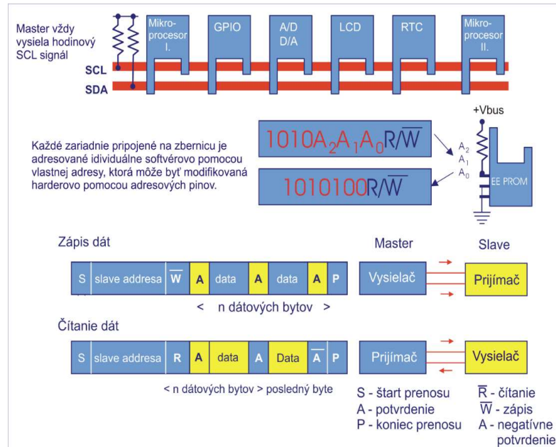
Obr. 87 Princíp komunikácie na I2C zbernici
