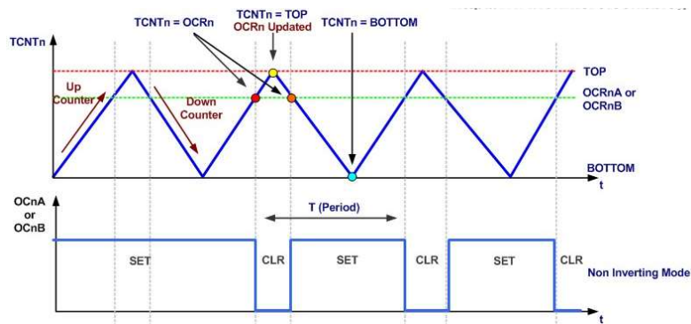
Obr. 71 Příklad časového priebehu zmeny výstupu OC0A v režime Phase Correct PWM
