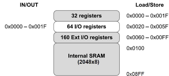
Obr. 37 Adresový priestor dátovej pamäte ATmega328P
