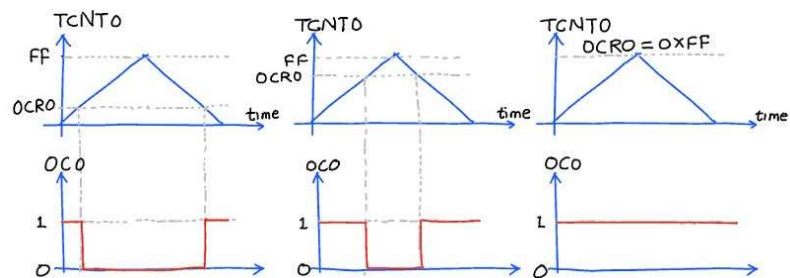
Obr. 68 Jednoduché znázornenie neinvertujúceho Phase Correct PWM signálu
