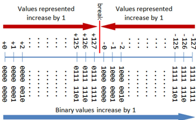
Obr. 16 Kódovanie binárnych čísel znamienkovým bitom
