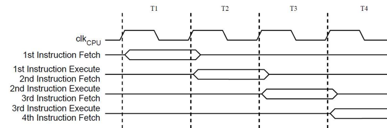
Obr. 23 Paralelné vykonávanie inštrukcií
