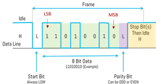
Obr. 80 Formát dát sériového prenosu - Frame format
