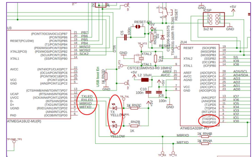
Obr. 82 Zapojenie vývodov RXD, TXD (ATmega328P) s prevodníkom Serial/USB (ATmega16)
