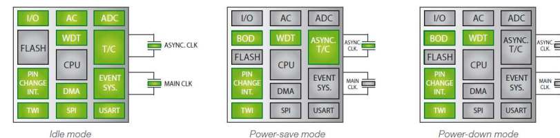
Obr. 40 Grafické znázornenie niektorých napájacích režimov MCU
