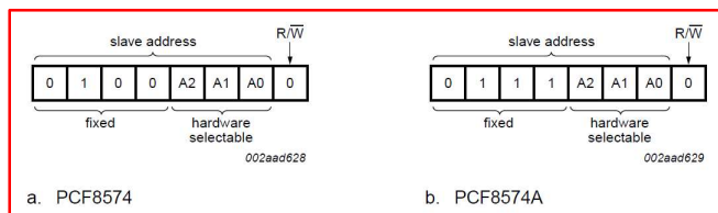
Obr. 101 Slave adresa obvodov PCF8574/74A
