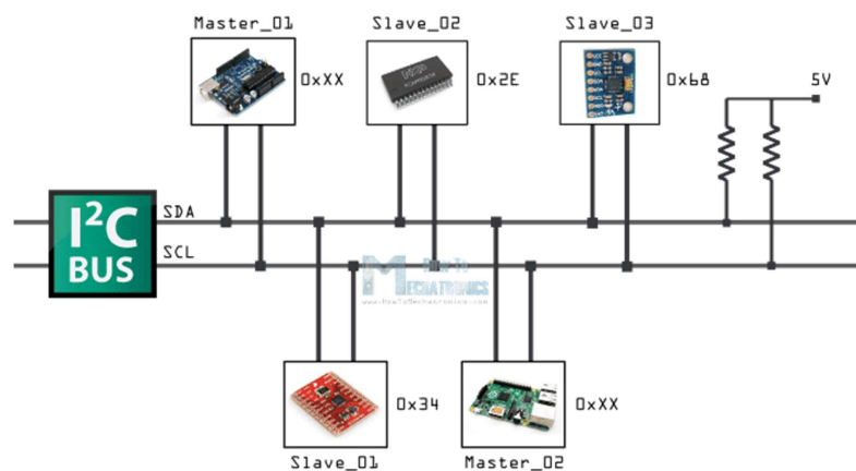
Obr. 83 Príklad pripojenia zariadení k I2C zbernici
