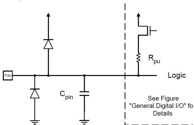
Obr. 49 Schéma vstupno-výstupného vývodu
