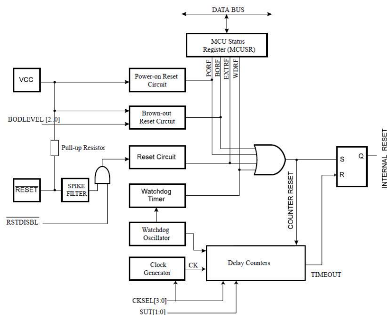
Obr. 41 Logika resetovacieho signálu ATmega328P
