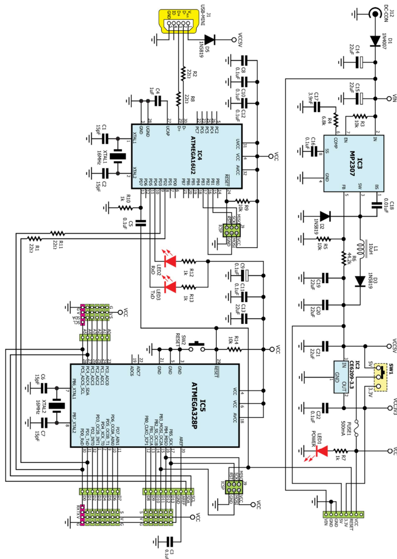
Obr. 92 Elektrická schéma zapojenia vývojovej dosky Arduino UNO
