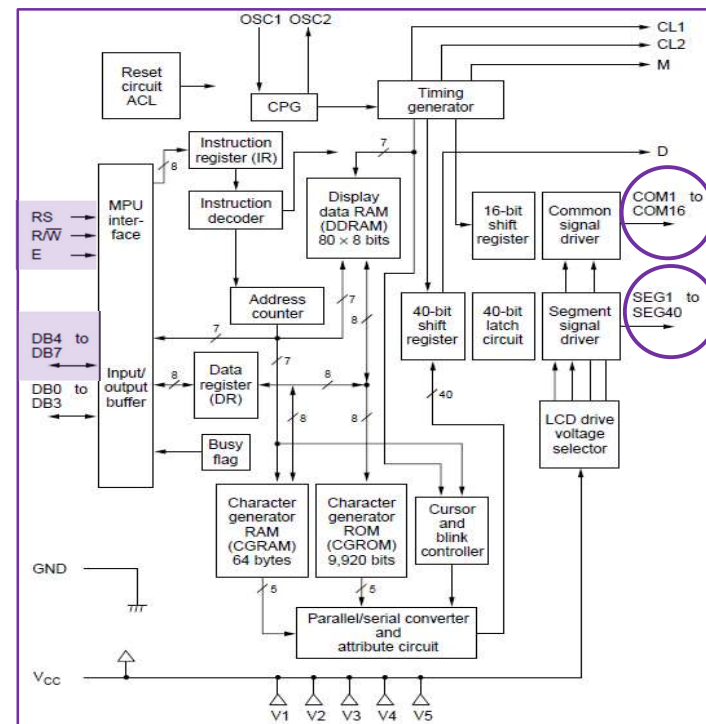
Obr. 96 Bloková schéma radiča HD44780U
