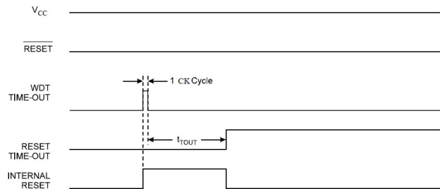
Obr. 45 Časový priebeh WatchDog System Reset
