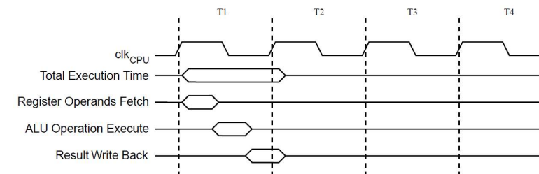
Obr. 24 Perióda vykonávania operácie v ALU
