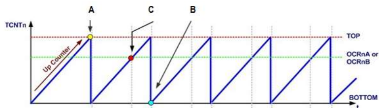
Obr. 59 Stavy počítadla TCNT0 a smer počítania
